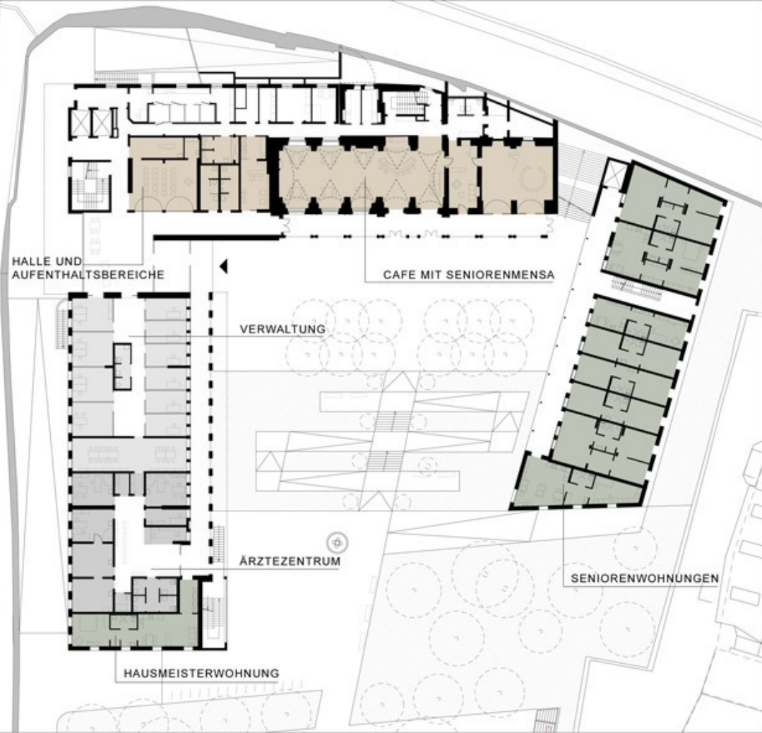
ERDGESCHOSS
