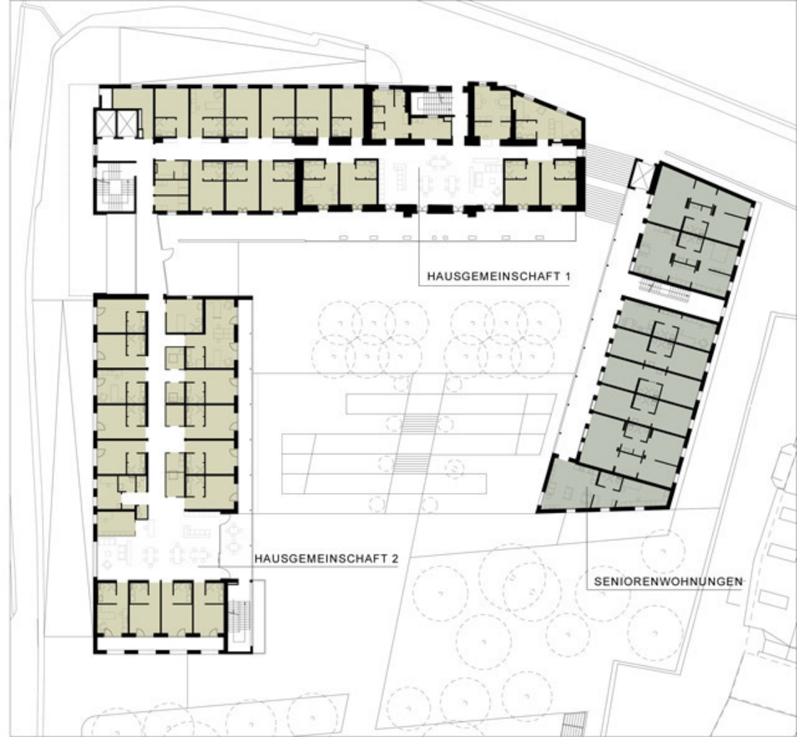
OBERGESCHOSS
