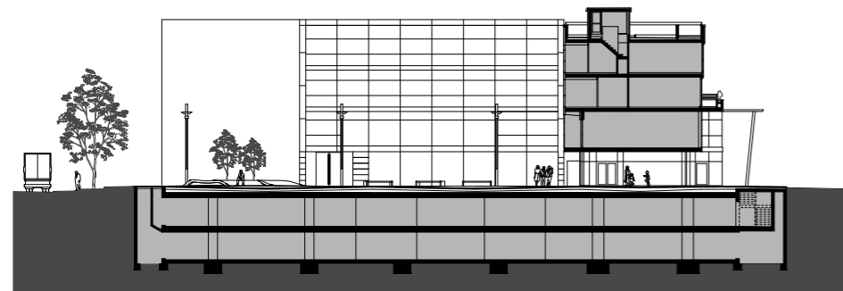
SCHNITT A-A
