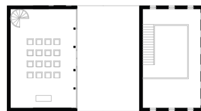
Grundriss Obergeschoss
