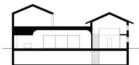
Schnitt
