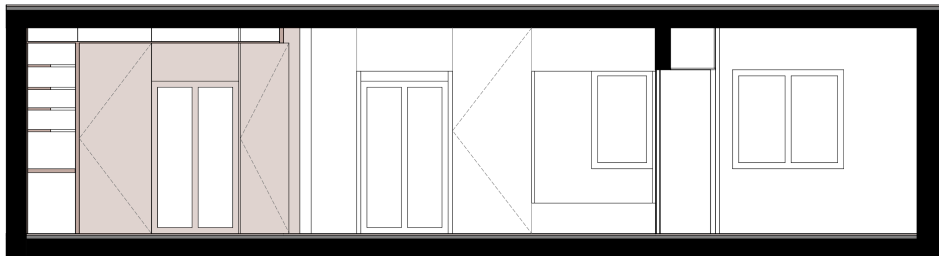
SEZIONE A-A
